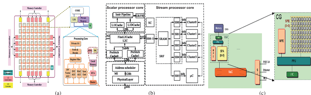
图 3 (网络版彩图) 国产众核处理器
